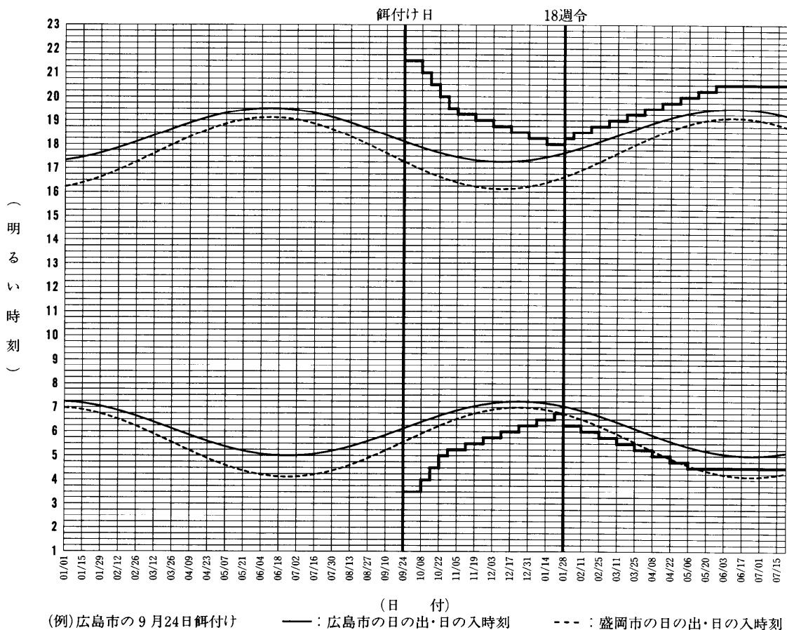
図3 オープン鶏舎での8月19日から2月14日までにつ化した鶏群の点灯プログラム例
